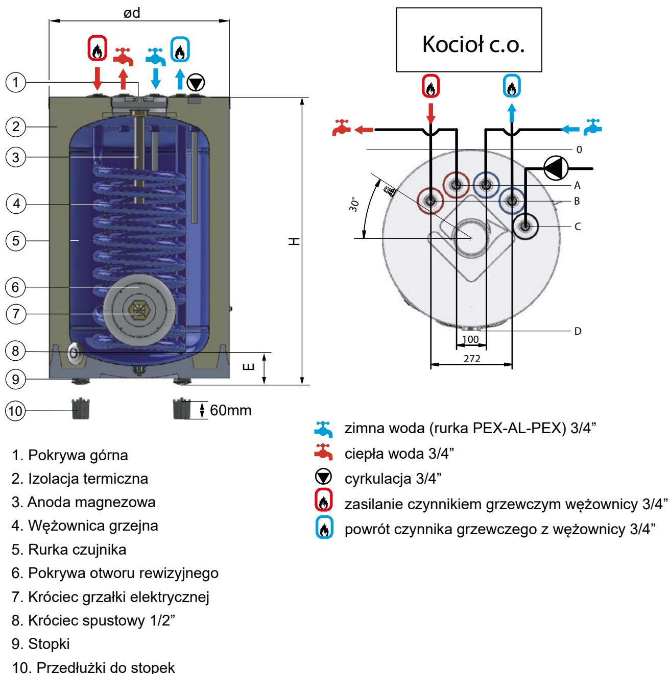
Rys. 1 – Budowa i wymiary podgrzewacza
