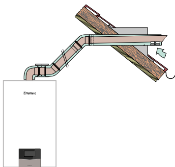
Poziome odprowadzanie spalin przez dach (przewód koncentryczny)
