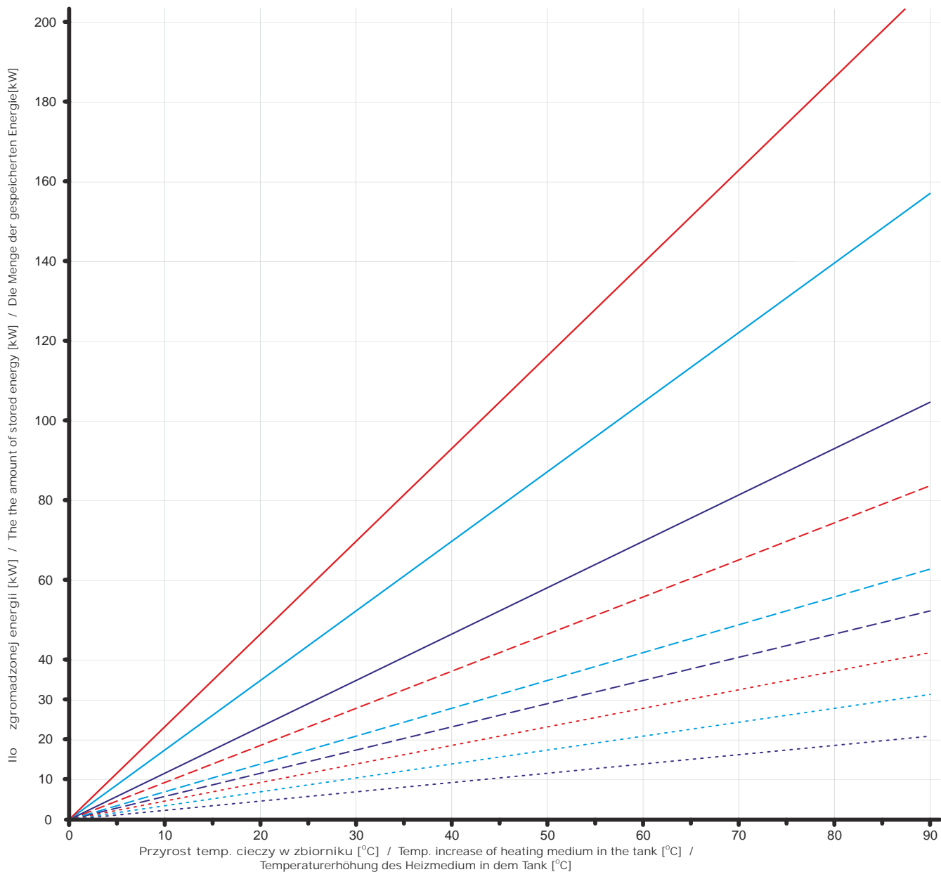
WYKRES KUMULOWANIA ENERGII PRZEZ ZBIORNIKI BUFOROWE Ciecz - woda,
