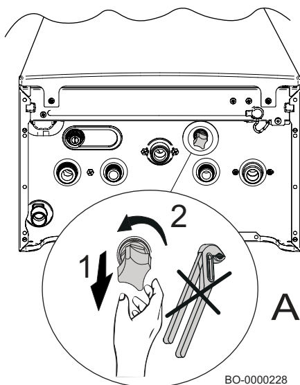
Rys.8 Napełnienie instalacji
