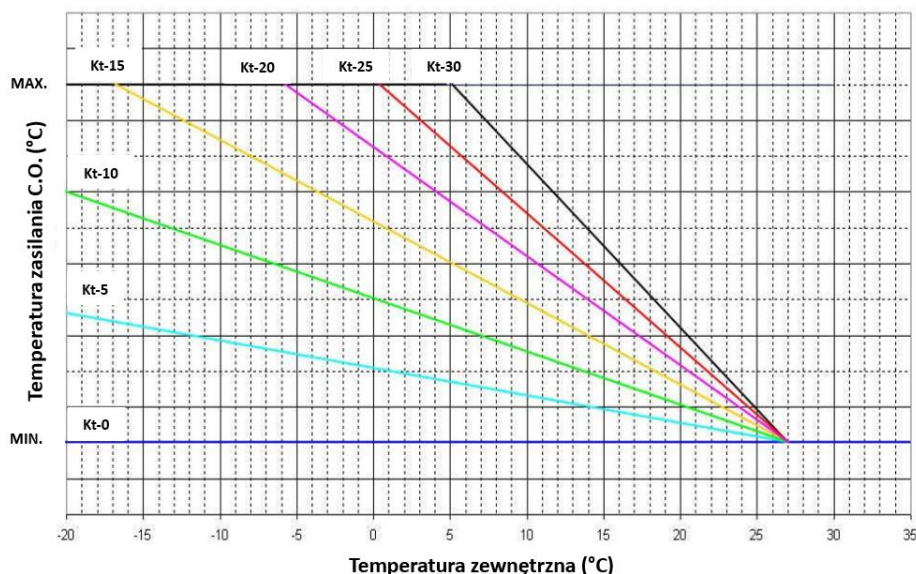
Rys.2.4.2.1 Wykres krzywych grzewczych
