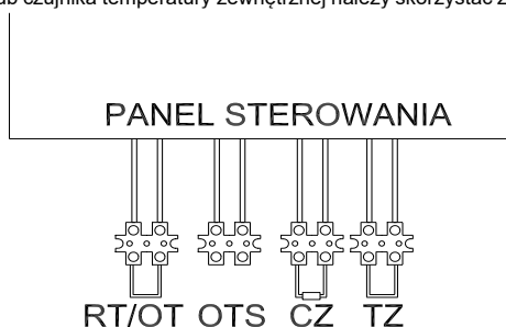
Rys.3.9.1 Płytki sterownika
